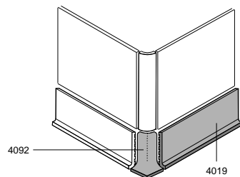
4092 | CANTO DE RODAPÉ ARREDONDADO ÂNGULO EXTERNO Rounded Baseboard Corner Outside Angle Ângulo de Zócalo Redondeado Ângulo Externo (30 X 100 X 30 mm)
