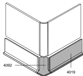
4019 | RODAPÉ PARTE SUPERIOR 90° Baseboard Upper Part 90° Zócalo Parte Superior 90° (240 X 100 X 9 mm)
